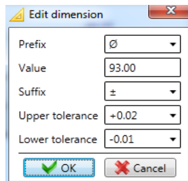
Figure 4 : Cotation
