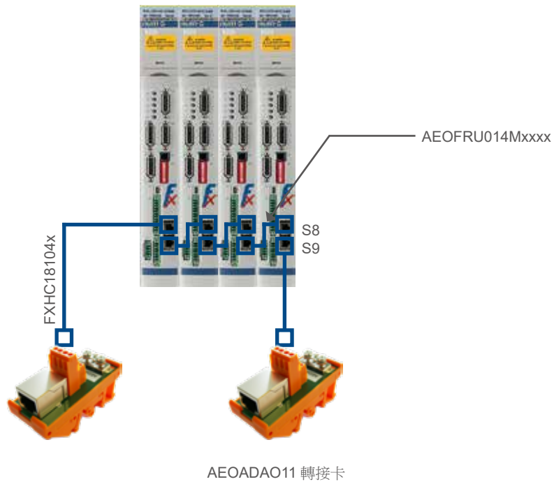
帶 NUM-STOX 的 NUMDrive X
