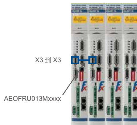
帶 Tandem 的 NUMDrive X
