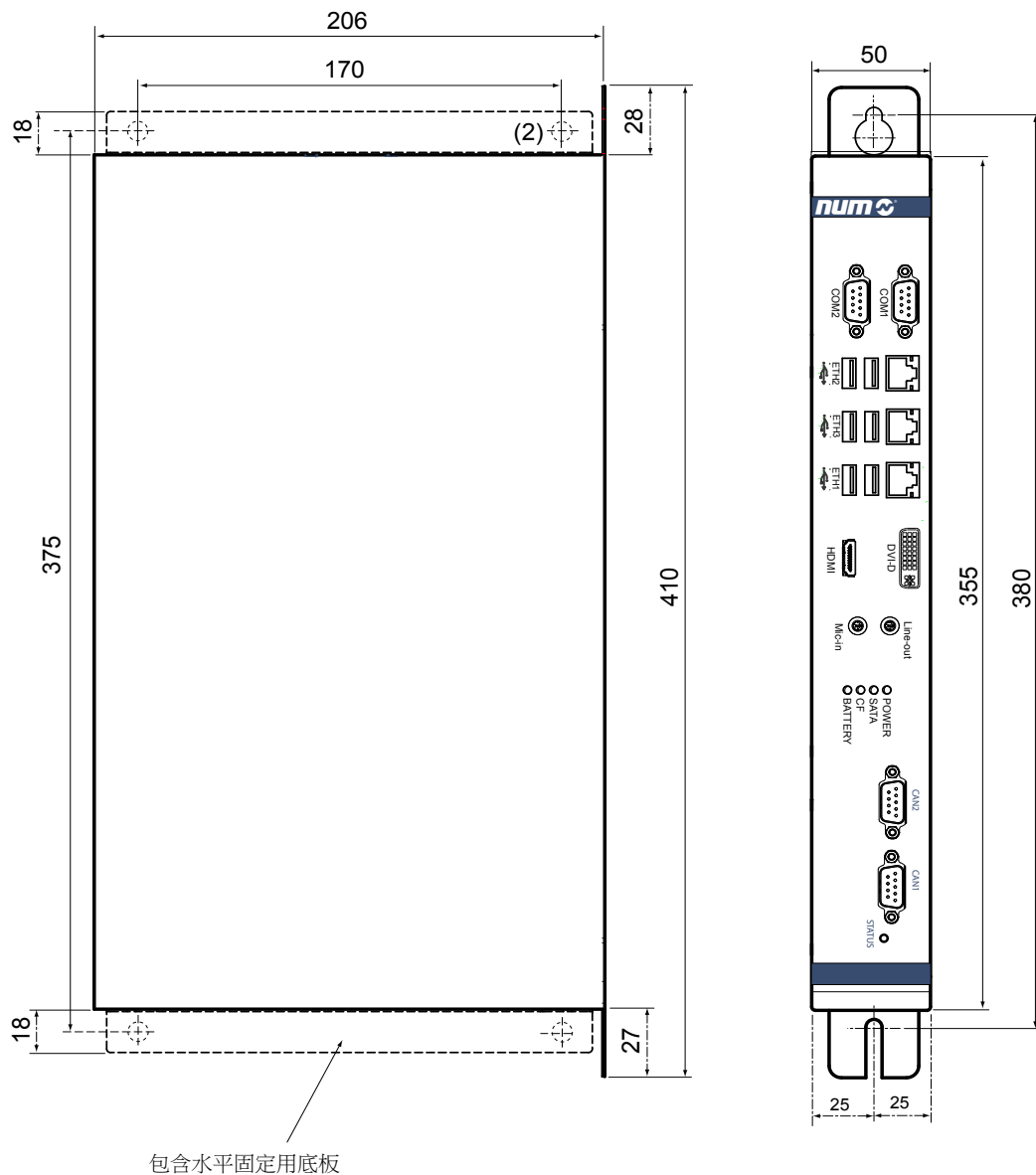
NUM 工業盒式 PC P2 簡圖 (FXPC004NN2SxR20)
