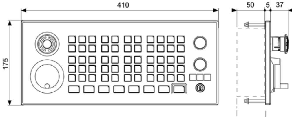
MP04-H 和 MP04-W 機床面板簡圖
