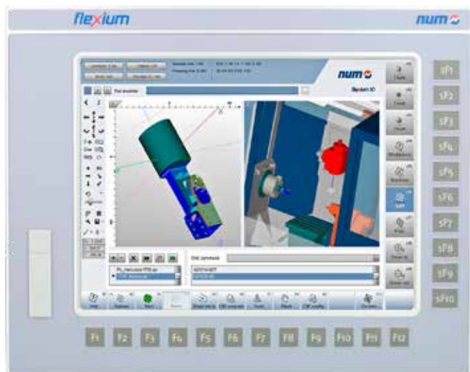
帶 22 個功能鍵的面板
