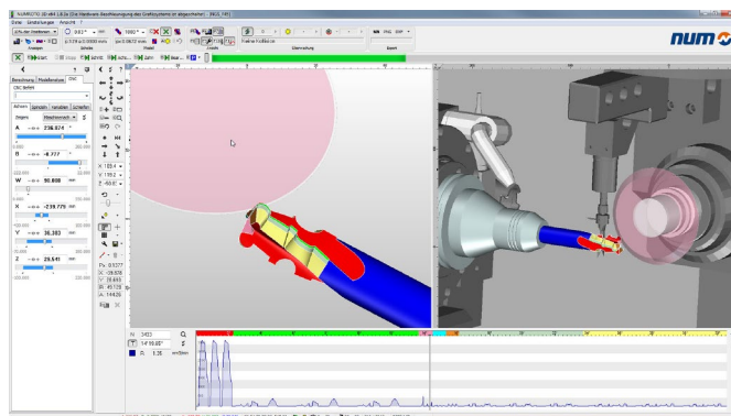
Beispiel einer NUMROTO 3D-Simulation.
